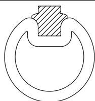
Ressort d'ajustage pour axe tubulaire 1"
