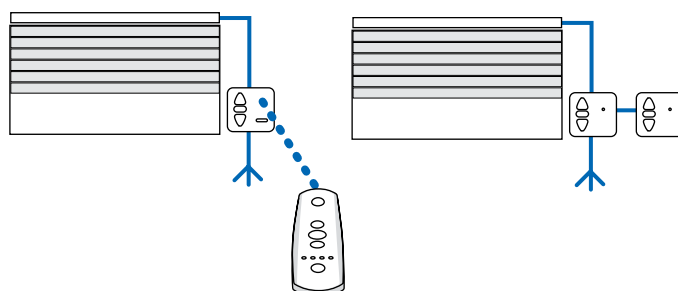
Centralis Uno RTS Commande filaire permettant la centralisation sans fil par radio
